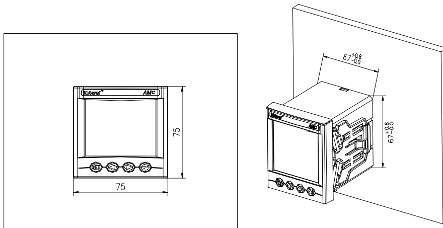
图 4 AMC72 安装尺寸
