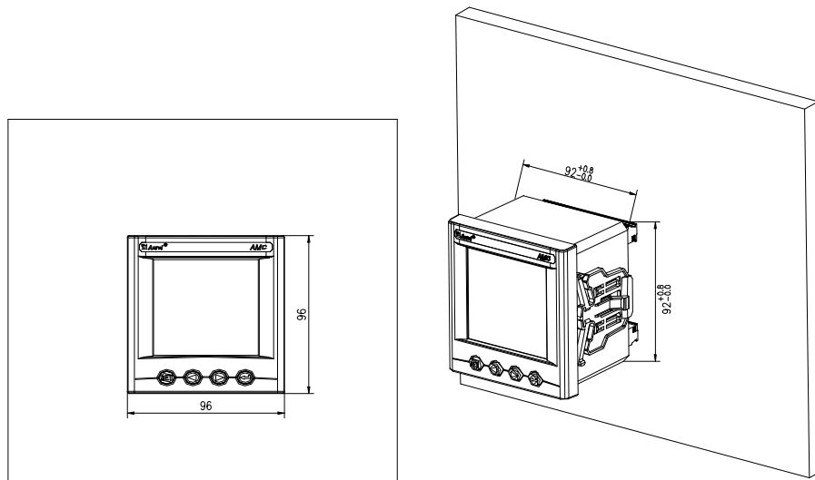
图 5 AMC96 安装尺寸
