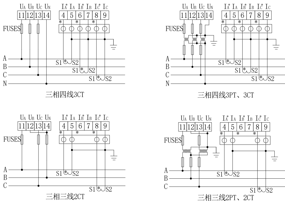
图10 仪表信号接线示意图
